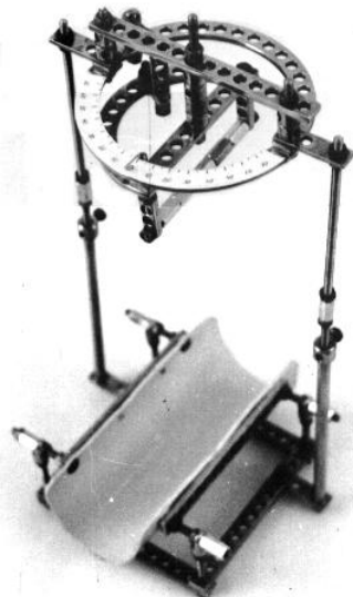
Рис. 2. Тренажер-ротаметр
