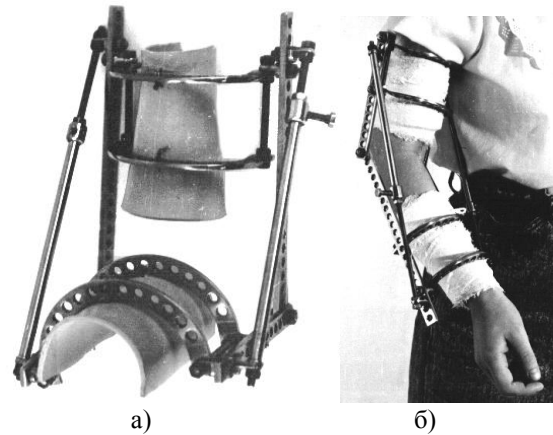
Рис. 4. Механическое устройство для разработки контрактур локтевого сустава: а) общий вид, б) в рабочем положении.
